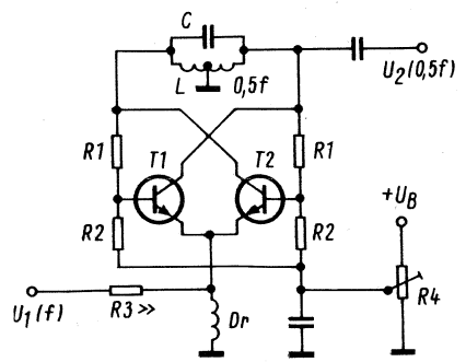
Bild 6. Frequenzteiler in Gegentaktschaltung
