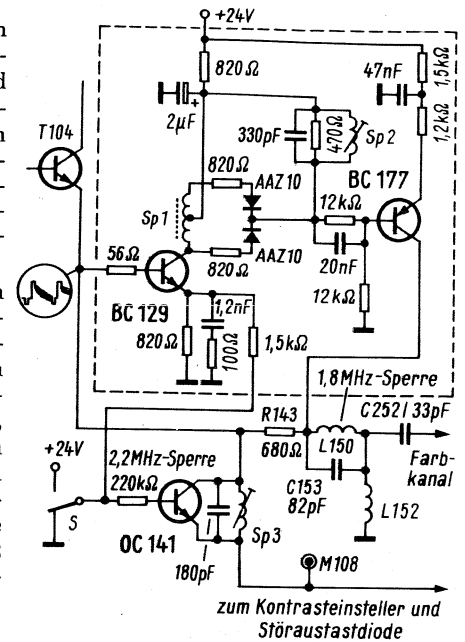
Bild 8. Farbträgerfrequenzverdoppler in einem Versuchsgerät
