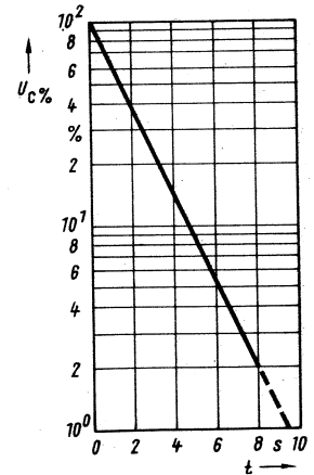
Linear-logarithmisch geteilte Achsen
