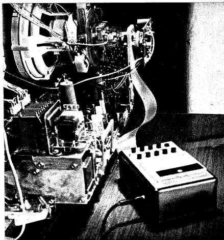
Das Bildröhren-Meßgerät der Firma Ing. Ed. Coßmann, angeschlossen an ein Fernsehgerät
