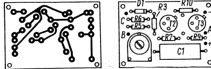
Bild 4. Druckplatine für die Schaltung von Bild 2
