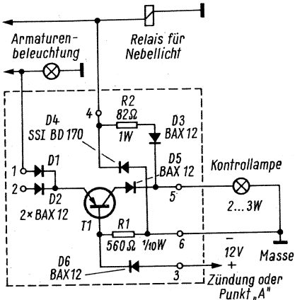
Bild 1. Einfache Elektronik zur Scheinwerferkontrolle
