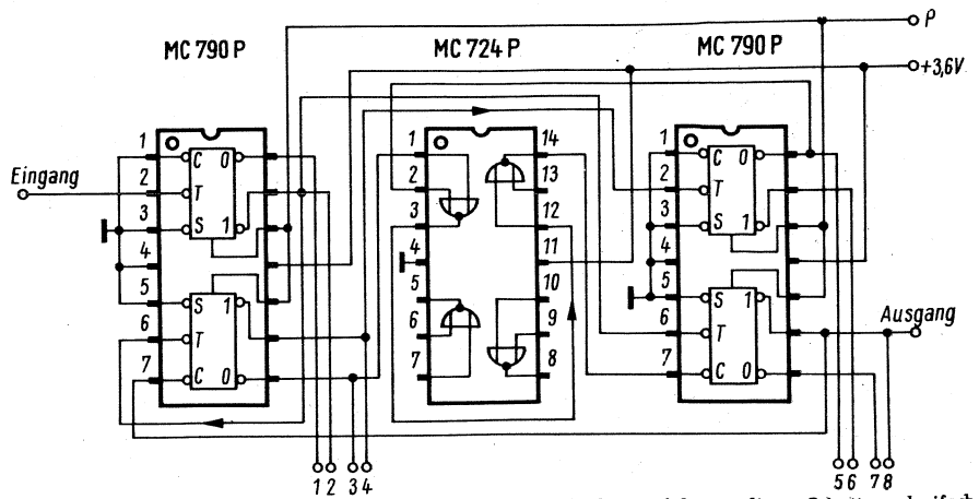
Bild 8. Verdrahtung der integrierten Schaltungen für eine Dekade. Ausführung dieser Schaltung dreifach
