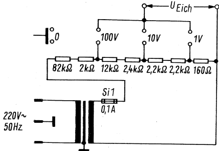
Die Schaltung des Eichspannungsteilers
