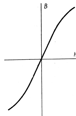
Rechts: Bild 6. Resultierende Kennlinie bei Hf-Vormagnetisierung
