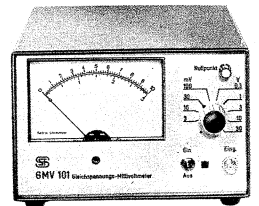
GMV 101 Gleichspannungs-Millivoltmeter
