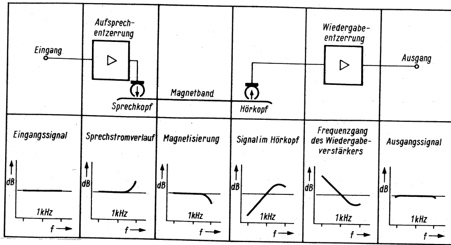
Bild 7. Entzerrung des Signals bei Aufnahme und Wiedergabe
