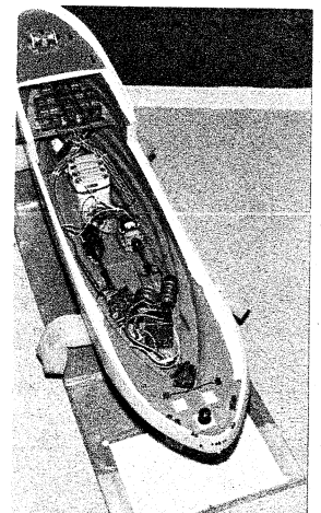
Rechts: Bild 10. Innenansicht des Modellbootes bei herausgenommenem Antriebsakkumulator
