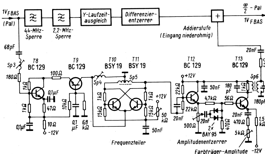
Bild 7. Gerät zur Farbträgerfrequenzhalbierung
