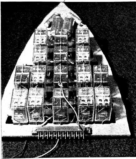
Bild 11. Nahansicht des Relaischaltteils
