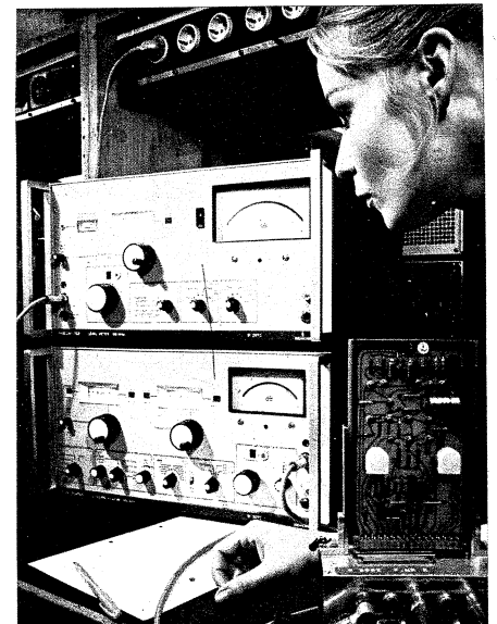
Dieser Pegelmeßplatz besteht aus dem Pegelsender W 2072 und dem Pegelmesser D 2072
