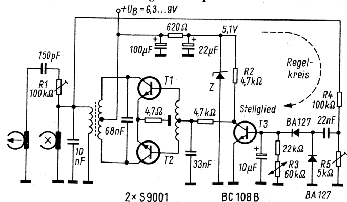
Hf-Oszillator des Grundig-Tonbandgerätes TK 3200 mit Spannungs-, Temperatur- und Amplitudenstabilisierung
