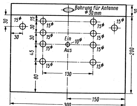
Bild 9. Maße des Sendergehäuses
